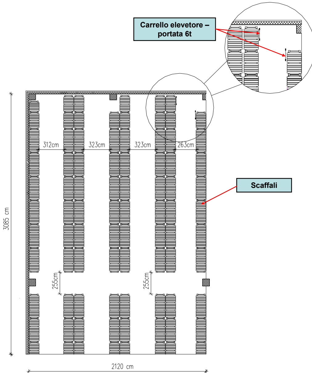
Figura B.10. Campo di pavimentazione n°1 del blocco 2: disposizione dei carichi considerati nell'analisi numerica.
