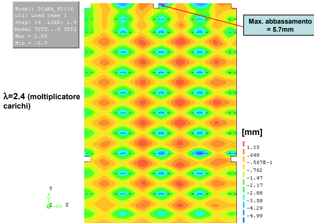
Figura B.11. Campo di pavimentazione n°1: contour degli spostamenti verticali presenti nella pavimentazione in corrispondenza del carico massimo raggiunto ( \lambda=2.4 ).
