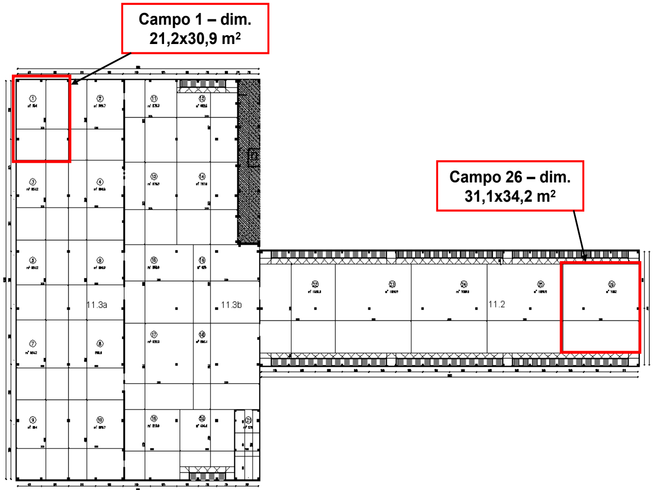
Figura B.5. Pianta della pavimentazione oggetto studio; in evidenza il campo di pavimentazione considerato nell’ambito dello studio numerico svolto.
