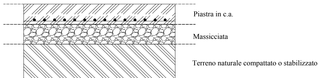
Figura 3.2. Sottofondo costituito da terreno naturale.
