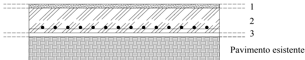
Figura 2.3. Pavimentazione su pavimentazione esistente.
