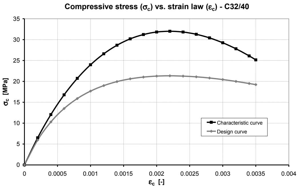
Figura A.1. Legame sforzo-deformazione a compressione del calcestruzzo fibrorinforzato.
