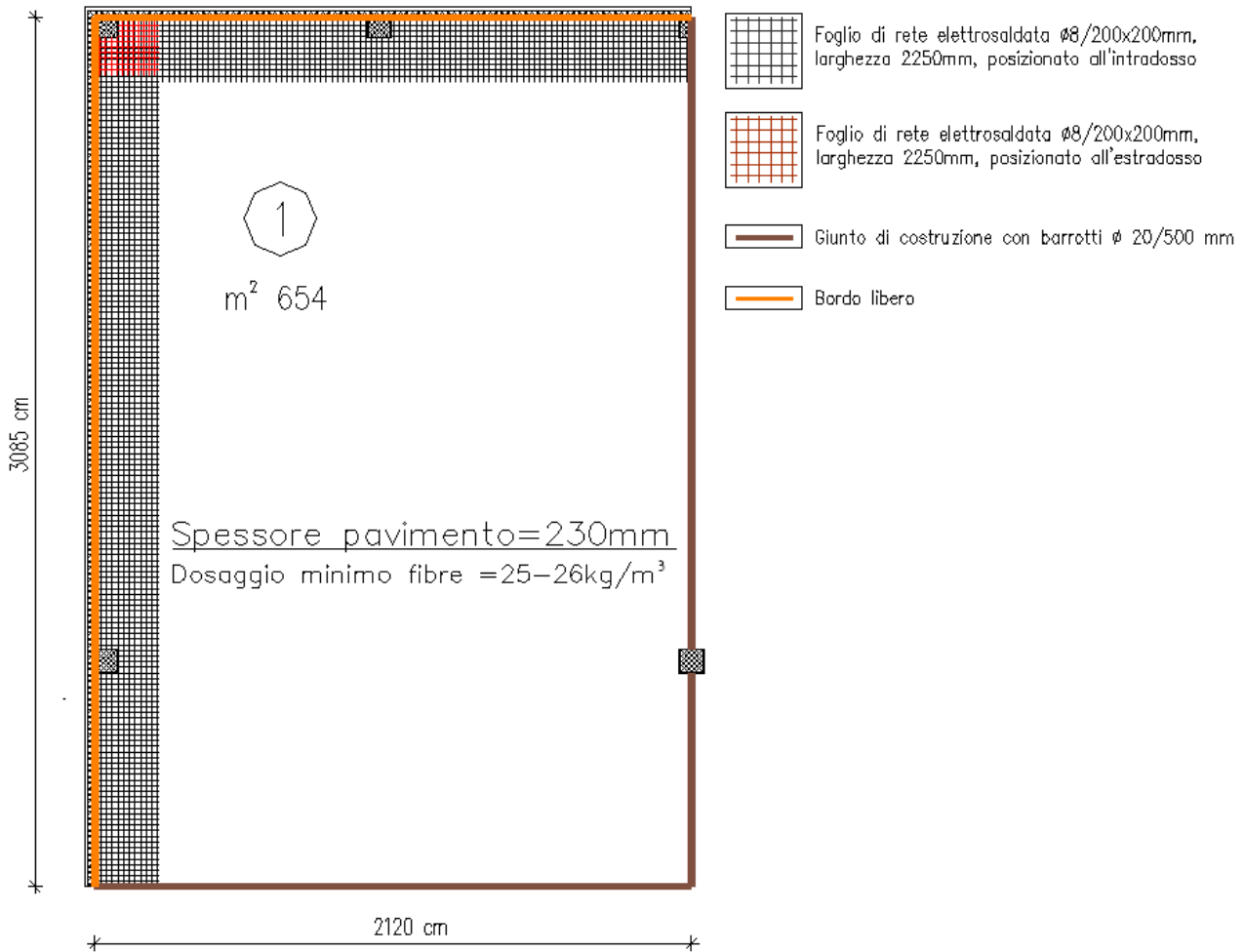
Figura B.6. Principali caratteristiche del campo di pavimentazione del Campo 1.
