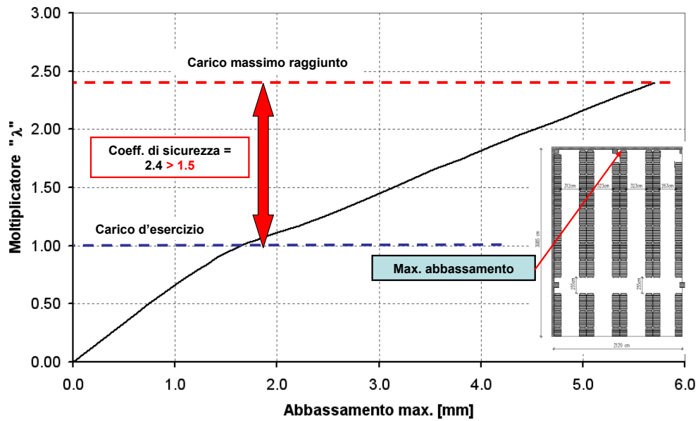
Figura B.12. Campo di pavimentazione n°1: andamento del carico in funzione dell'abbassamento massimo rilevato.
