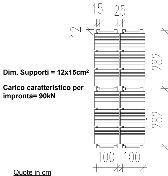
Figura B.9. Schematizzazione dei carichi applicati alla pavimentazione: supporti degli scaffali (a); singolo asse di carico del carrello elevatore (b).
