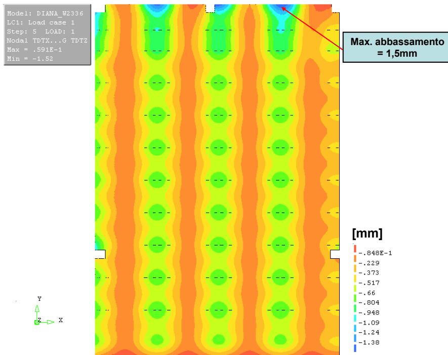
Figura B.15. Campo di pavimentazione n°1: contour degli spostamenti verticali presenti nella pavimentazione in corrispondenza del carico d’esercizio.
