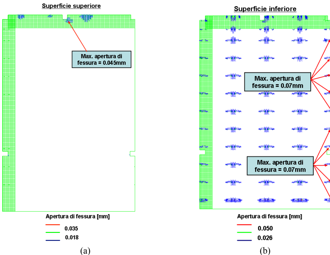
Figura B.16. Campo di pavimentazione n°1: contour delle fessure rilevate sulla superficie superiore (a) e inferiore (b) della pavimentazione, in corrispondenza del carico di esercizio.
