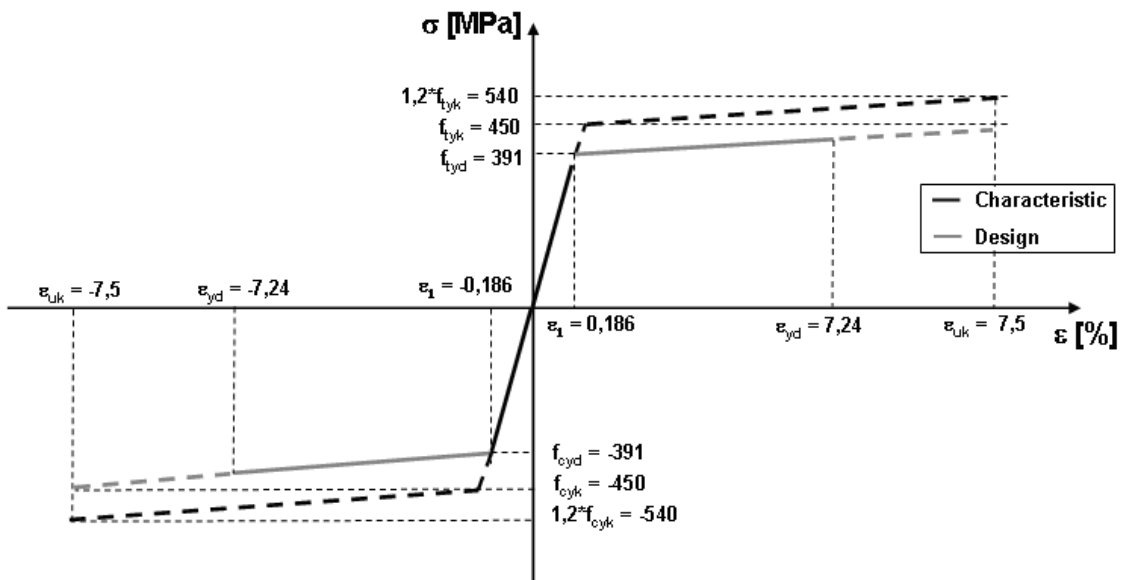
Figura B.4. Diagramma sforzo-deformazione adottato per l'acciaio per armature B450C.
