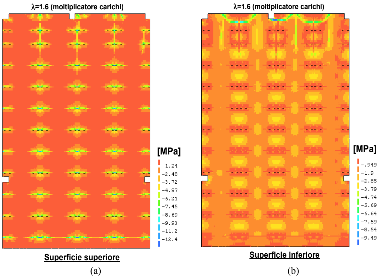
Figura B.13. Campo di pavimentazione n°1: contour degli sforzi principali minimi rilevati sulla superficie superiore (a) e inferiore (b) della pavimentazione in corrispondenza di un moltiplicatore dei carichi \lambda=1,6 .
