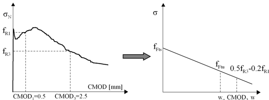
Figura B.2. Legge lineare impiegata per descrivere il comportamento a trazione post-fessura dell'SFRC.
