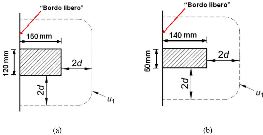
Figura B.14. Campo di pavimentazione n°1: perimetro di verifica “ u_1 ” (Eurocodice 2) considerato per i supporti degli scaffali (a) e per le ruote del carrello elevatore (b).
