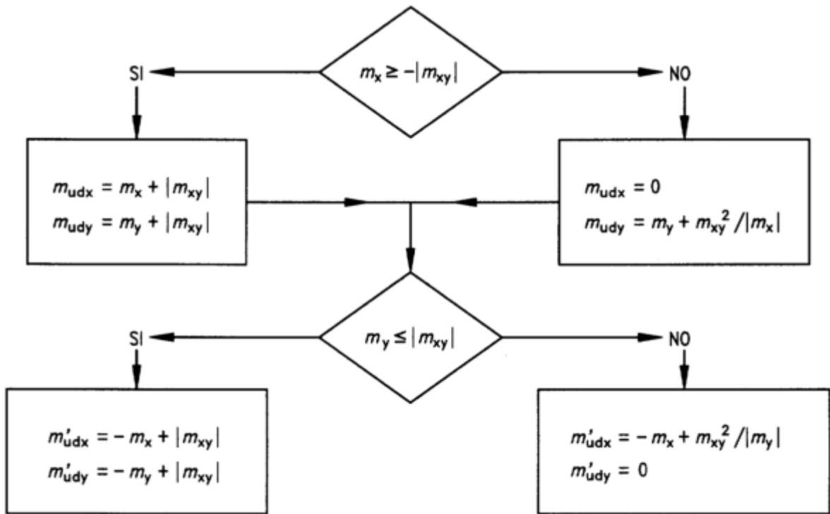
Figura A. 1. Diagramma di flusso per la valutazione di momenti sollecitanti m_{ud,x} ed m_{ud,y} .
