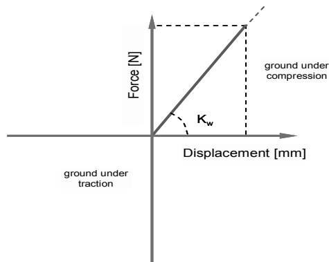
Figura B.8. Legame forza-spostamento assegnato agli elementi molla utilizzati per simulare il comportamento del sottofondo.
